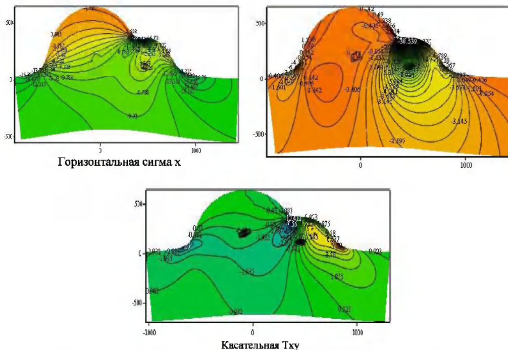
Рис. 2. Изолинии распределения напряжений / Fig.2. Isolines of stress distribution
