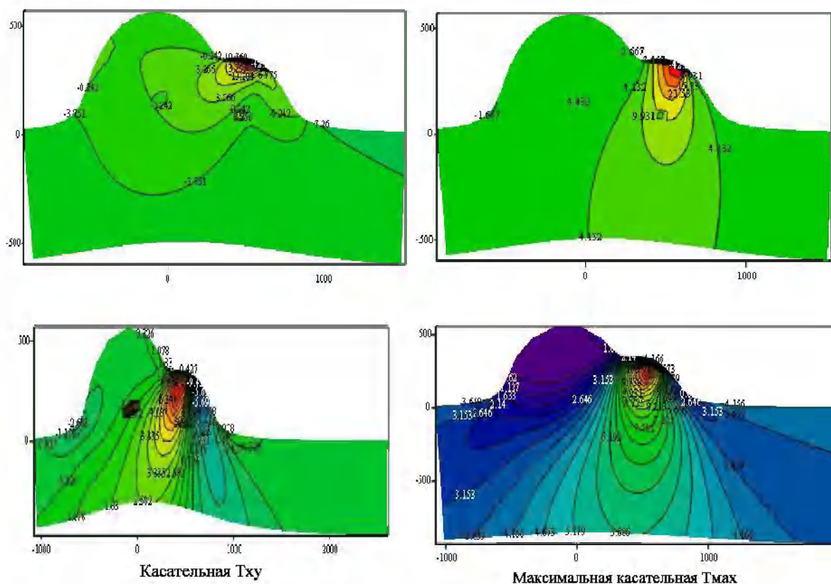
Рис. 3. Распределения напряжений от действия гравитационных сил / Fig.3. Stress distributions from the action of gravitational forces
